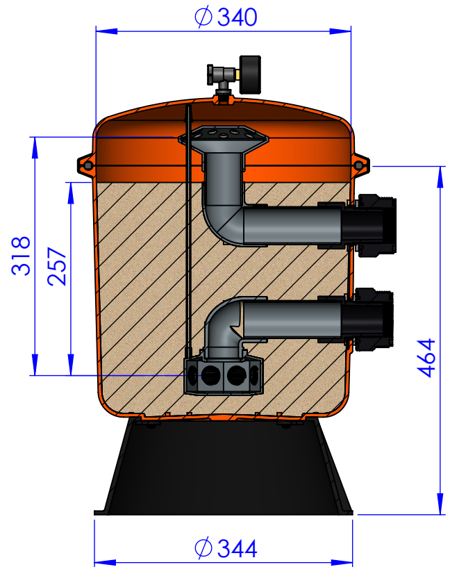
SECCIÓN A-A
