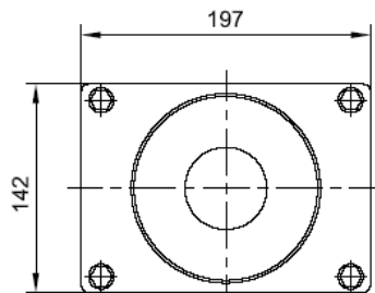
Схема крепления
