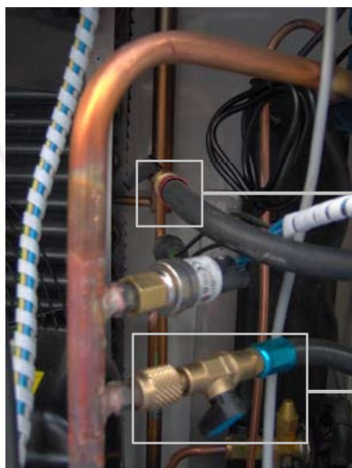
Клапан высокого давления
