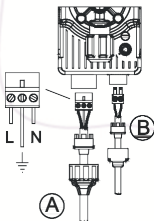
Рис. 12: Схема соединений Вход А = электропитание Вход В = датчика уровня реагента
