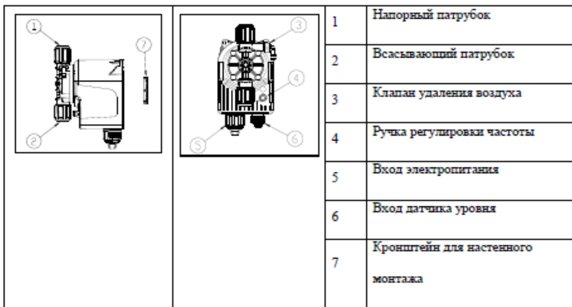
Рис.10. Составные части насоса
