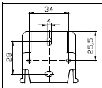
Рис.9 Шаблон для сверления
