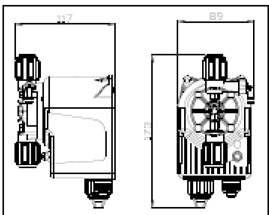
Рис.8 Габаритные размеры
