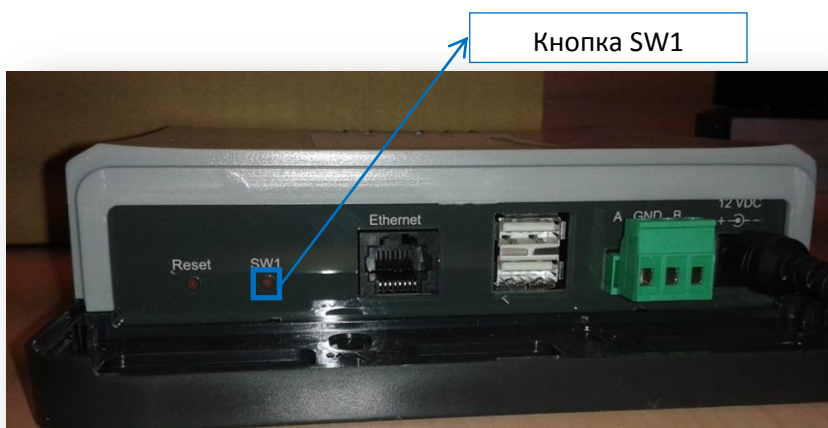
Рис 57: Задняя панель Connect Box
