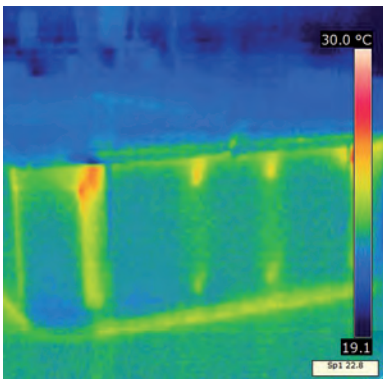
Испытание на утечку тепла, проведенное с системой изоляции «Nordic»
